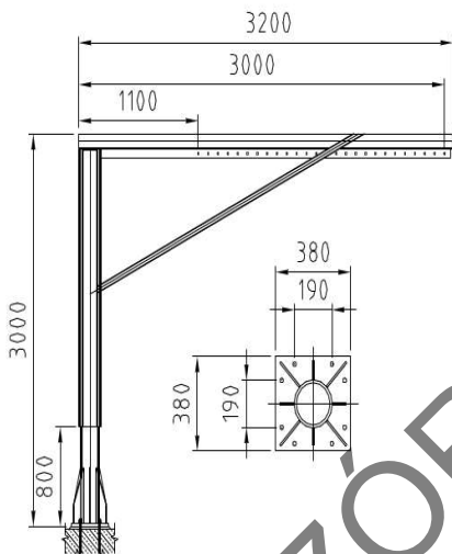
Rys nr 1 - Żuraw wraz z stopą mocowany do poziomego podłoża
