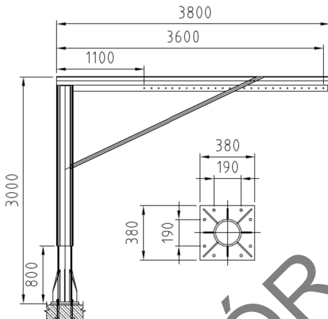
Rys nr 1 - Żuraw wraz z stopą mocowany do poziomego podłoża
