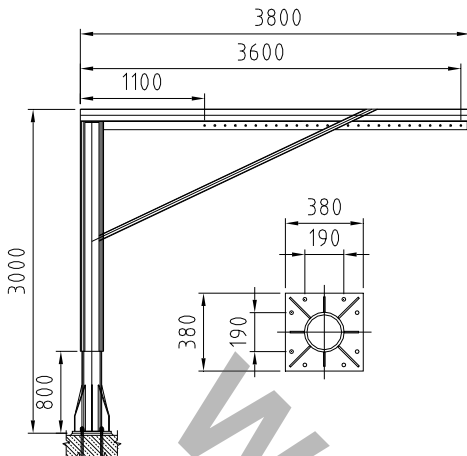
Rys nr 1 - Żuraw wraz z stopą mocowany do poziomego podłoża
