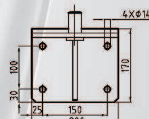
uchwyt górny
